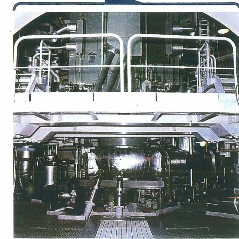
機器搬出入口から見る再循環ポンプ
