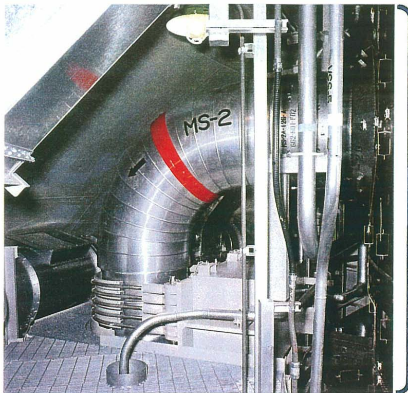
主蒸気ノズル廻りアクセスフロア
