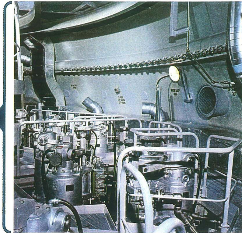
主蒸気逃がし安全弁メンテナンスフロア
