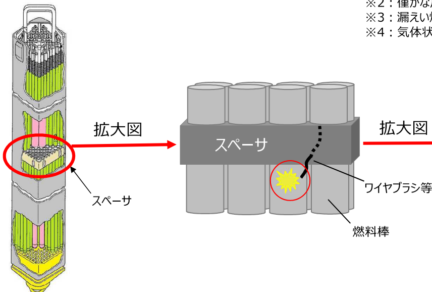
燃料集合体
