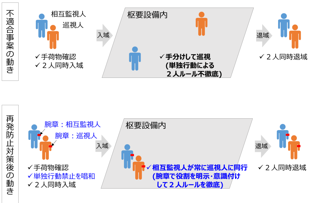
図2. 枢要設備における2人ルールのイメージ
