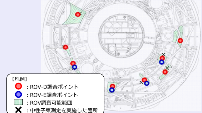
＜ROV-D,EによるPCV内部調査箇所＞
