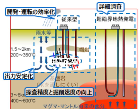
<地熱発電の技術開発・超臨界地熱発電>
