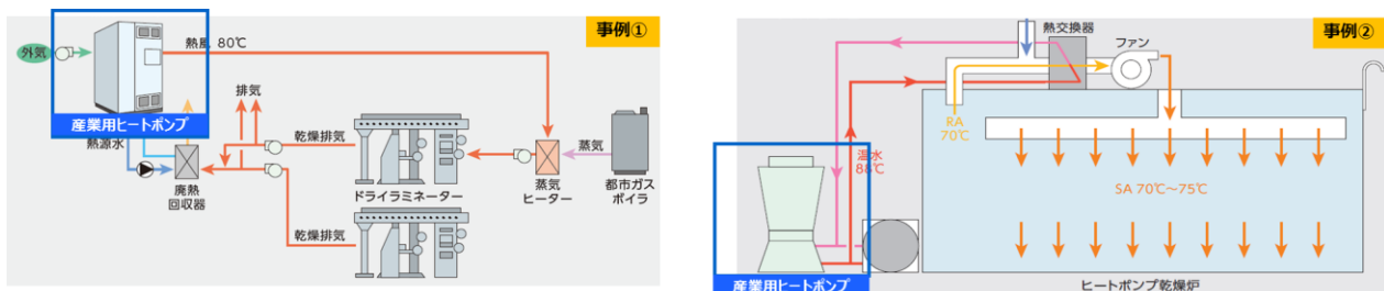
＜ヒートポンプ導入によるプロセス改善事例＞
