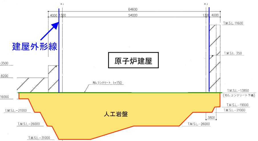
A-A断面図
