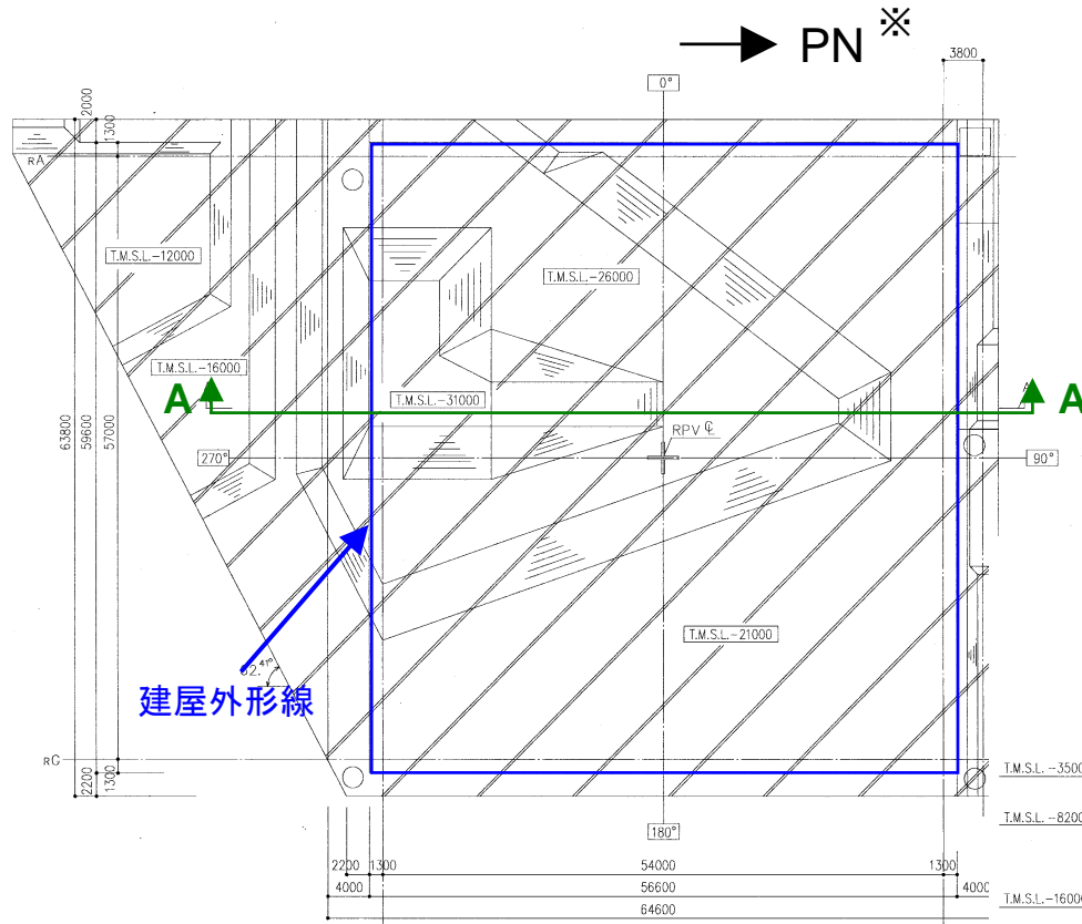
掘削床付図
