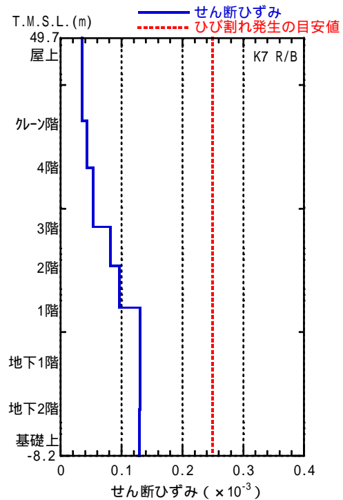
図 - 2 耐震壁のせん断ひずみ (東西方向)
