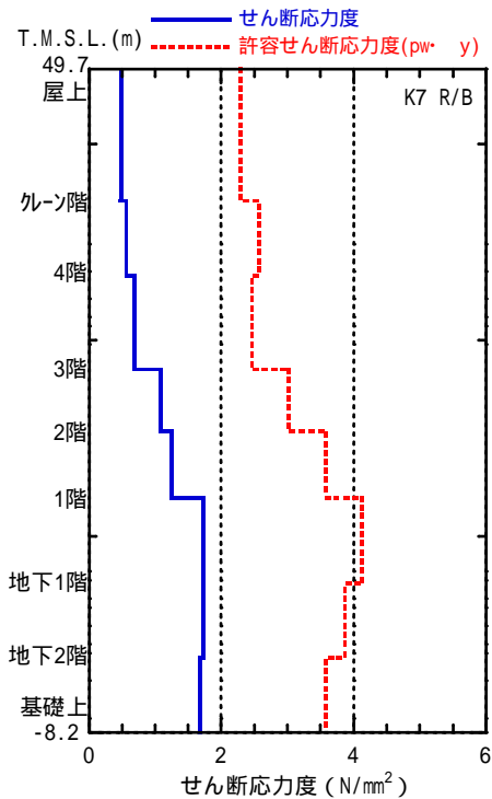
図 - 1 耐震壁のせん断応力度 (東西方向)
