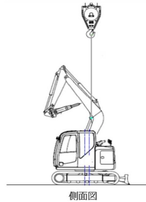
図1：本事象の誤った吊りに荷姿と作業再開時の吊り荷姿
