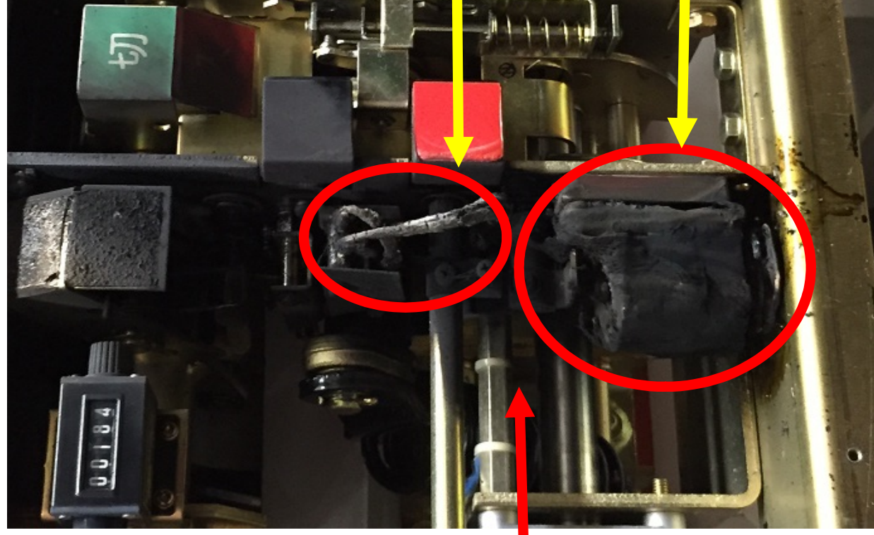
火災箇所(遮断器トリップコイルおよび電気コード被覆)拡大写真
